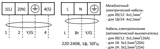
Внутренний блок моделей ASW-H09,12,18,24A4/FJ-R1DI
