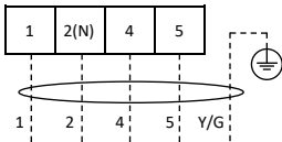
Наружный блок моделей AS-H07,09,12,18A4/FJ-R1
