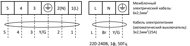
Внутренний блок моделей ASW-H09,12,18,24A4/FJ-R1DI
