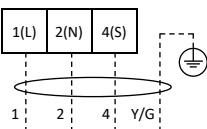
Наружный блок моделей AS-H09,12,18,24A4/FJ-R1DI
