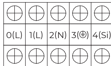
Клеммный терминал внутреннего блока
